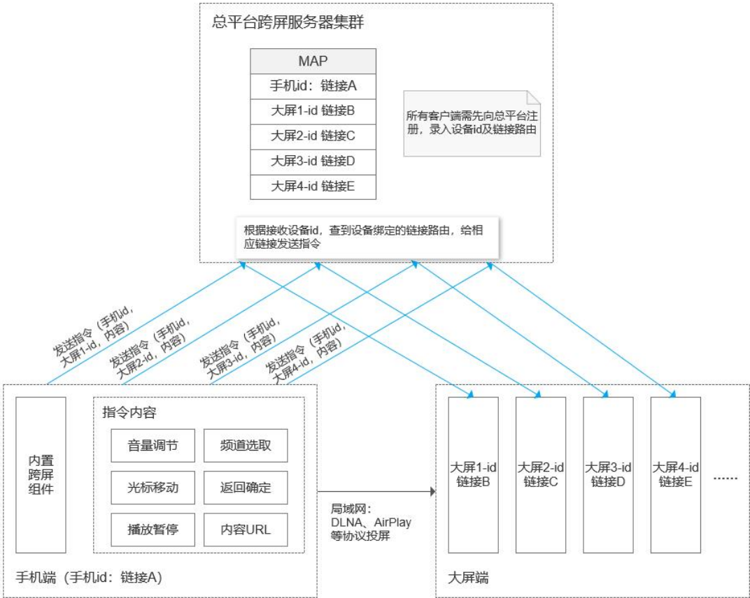
图 10 5G 频道总平台大小屏协同功能框图
